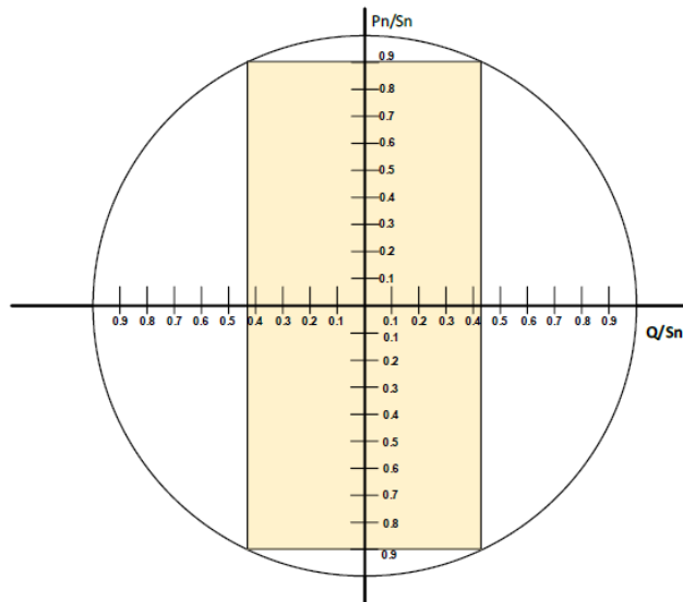
איור 4: גרף P/Q של המתקן
