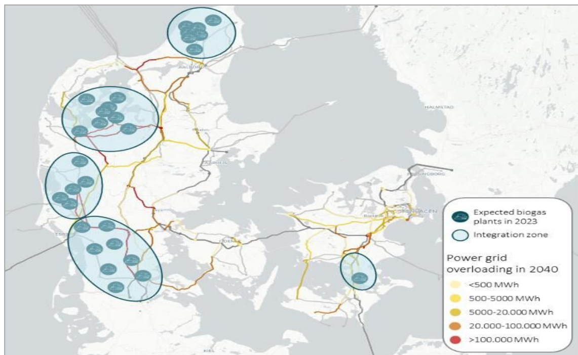
איור 7: שילוב מתקני ביוגז באזורים עם רשת עמוסה להפחתת עומסים
