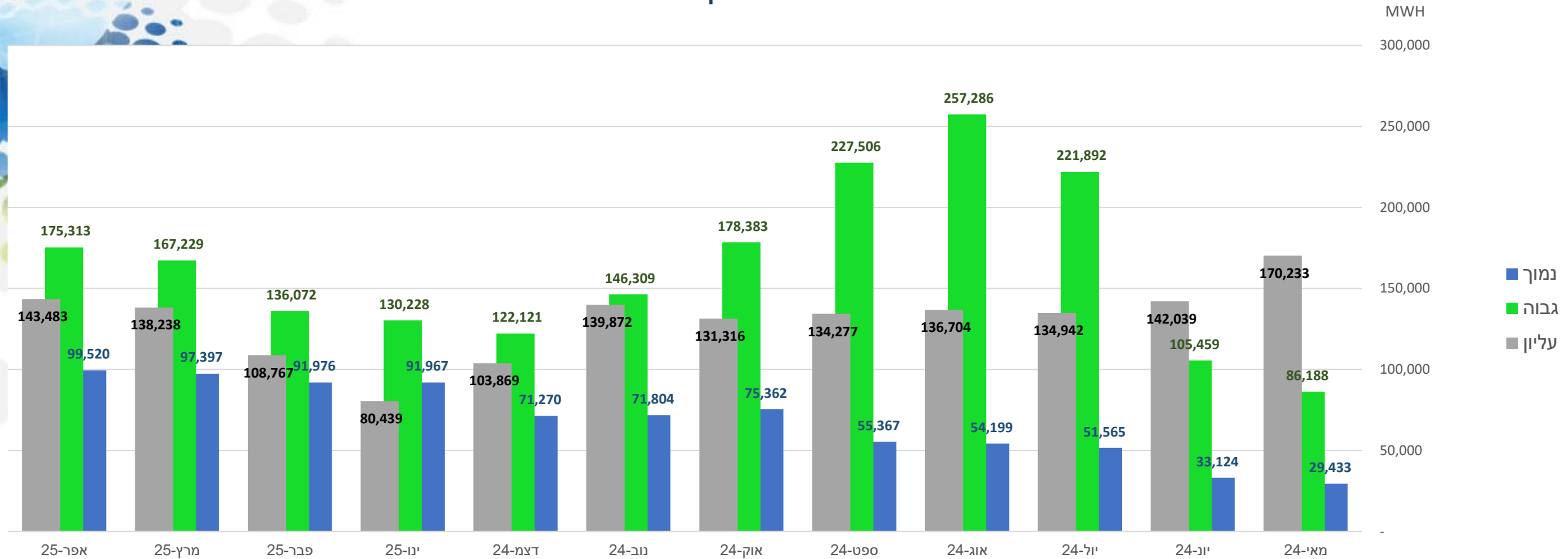
צריכה לפי רמות מתח - מספקים ווירטואליים
