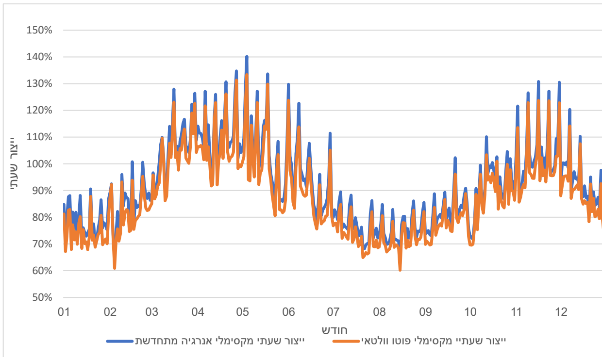
איור מס' 3.20: שיעור ייצור שעותי מקסימאלי בשנת 2030
