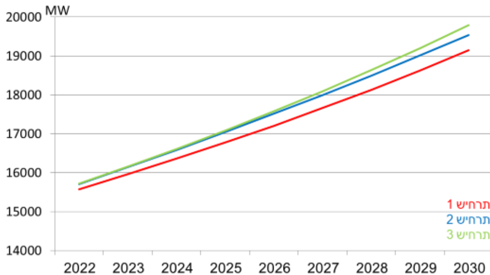
איור מס' 3.2: שיא קיץ (צהריים) לפי תרחישים שונים בשנים 2022 - 2030
