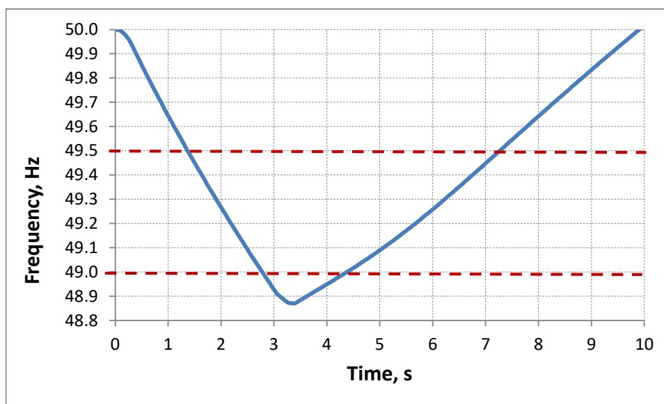
איור 4.4: התנהגות התדר באירוע הפסקה של 644 MW בשעה 11 בחודש אפריל בשנת 2023
