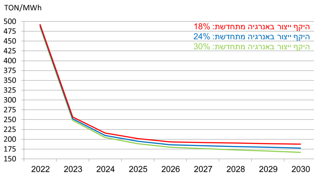
איור מס' 3.16: כמות סגולית של NO_x בשנים 2022 – 2030 (TON/MWh)
