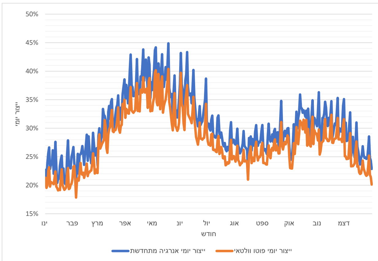
איור מס' 3.19: שיעור הייצור היומי בשנת 2030
