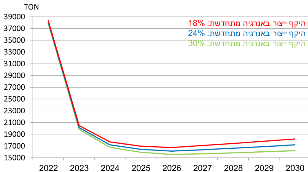
איור מס' 3.12: היקף NO_x בשנים 2022 – 2030 (TON)
