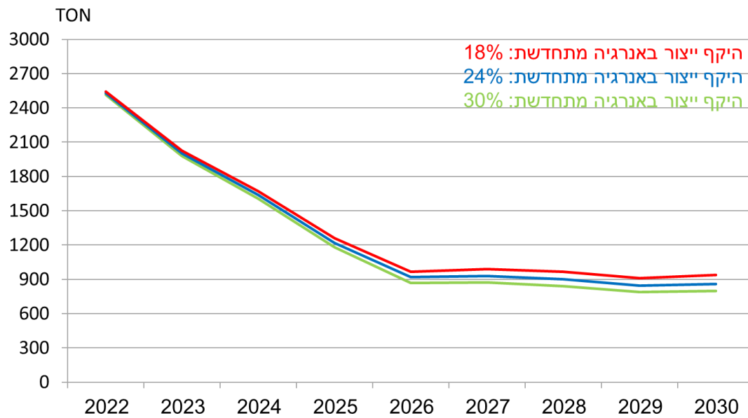
איור מס' 3.13: היקף חלקיקים בשנים 2022 – 2030 (TON)
