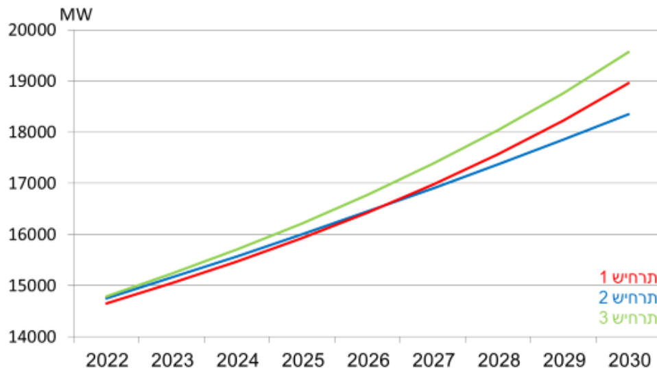
איור מס' 3.4: שיא חורף לפי תרחישים שונים בשנים 2022 - 2030
