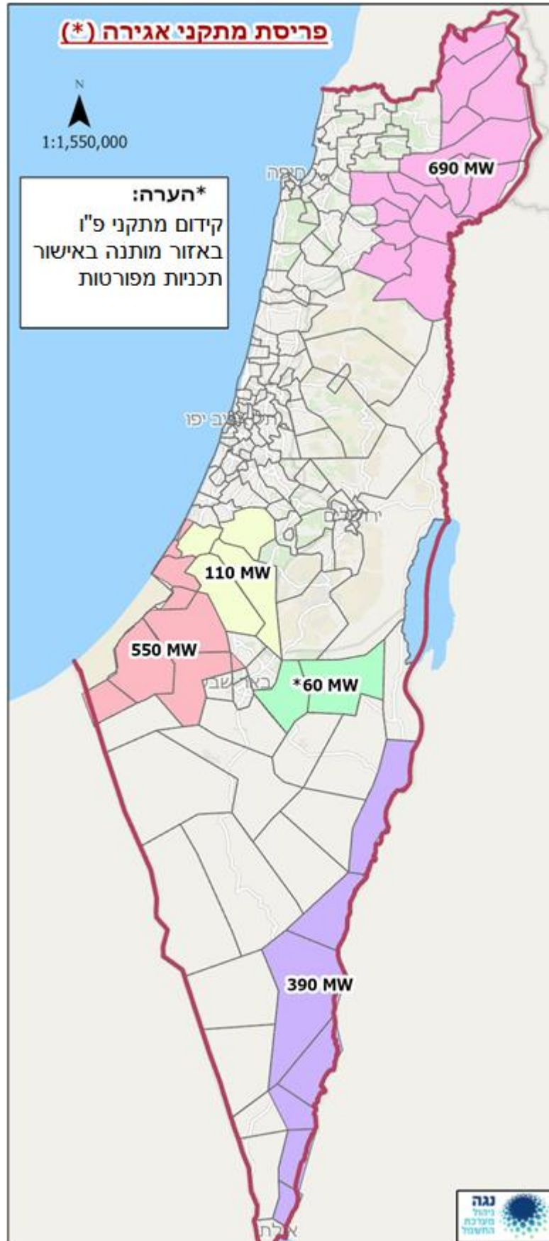
איור 5.26: פריסה של מתקני אגירת אנרגיה, בהספק מצרפי כ- 1800 מגוואט, שנקבעו ע"י תוכנית פיתוח מערכת היצור
