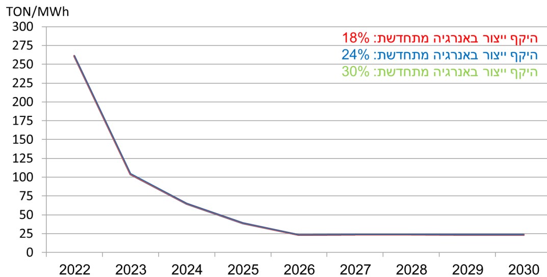
איור מס' 3.15: כמות סגולית של SO_2 בשנים 2022 – 2030 (TON/MWh)
