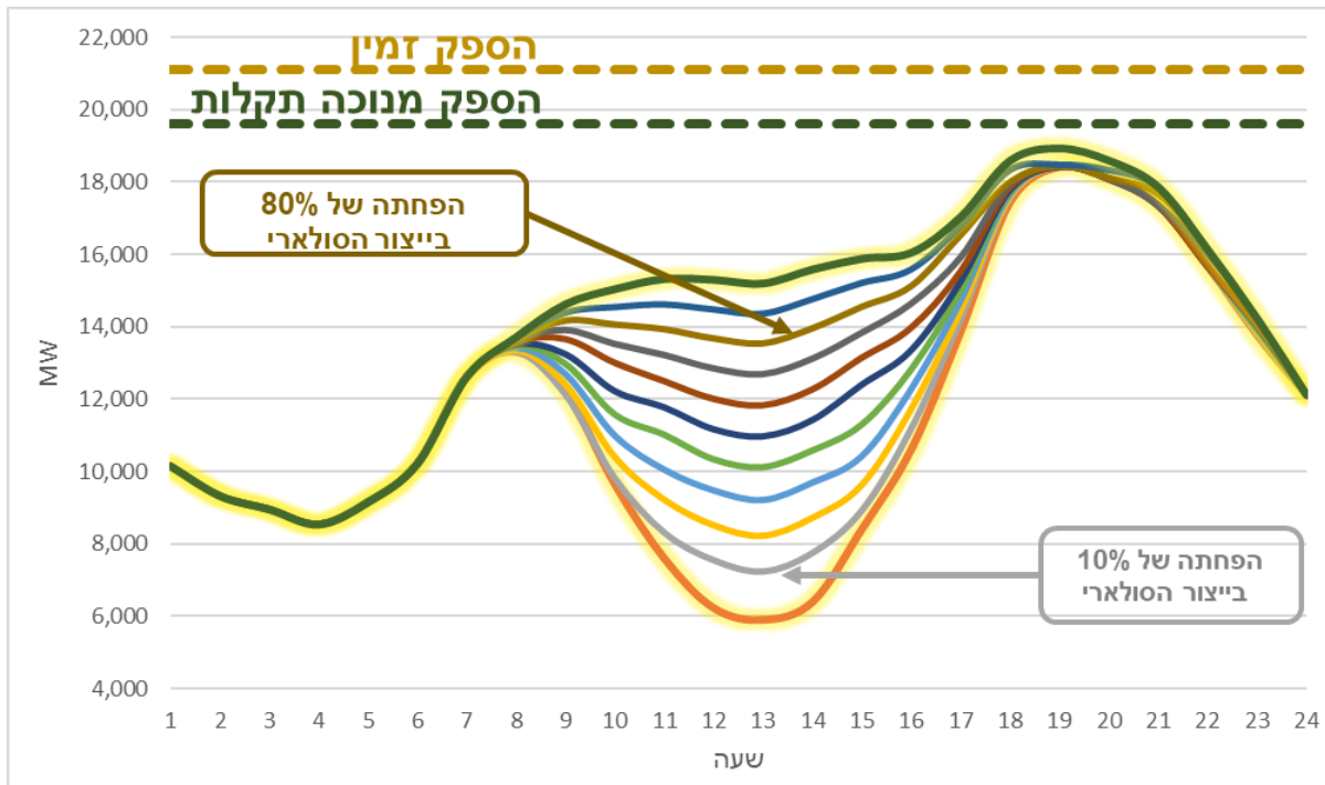
איור 3.21: עקומי ייצור שיורי ביום שיא חורף לפי תרחישי הפחתה שתוארו
